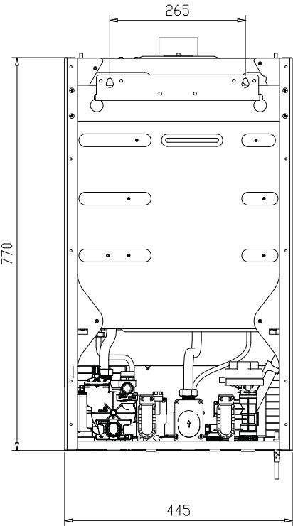
Чертеж размера котла
